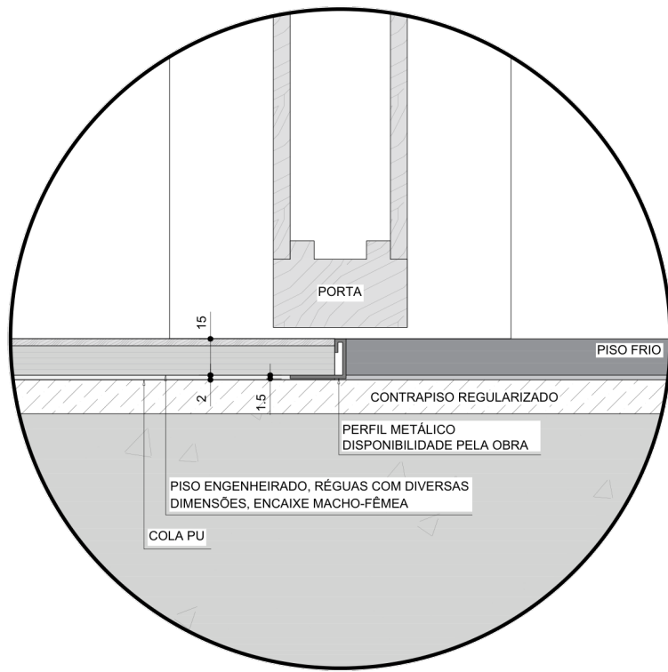
DET. 02 - TRANSIÇÃO DE PISO EM PERFIL METÁLICO ESC. 1:10
