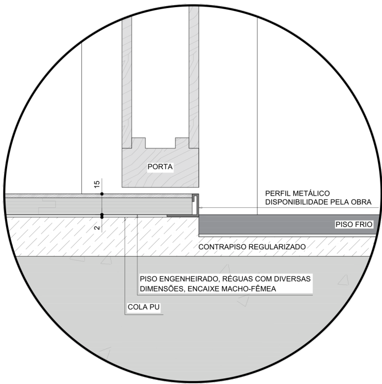
DET. 01 - TRANSIÇÃO DE PISO EM PERFIL METÁLICO COM DÉSNIVEL ESC. 1:10
